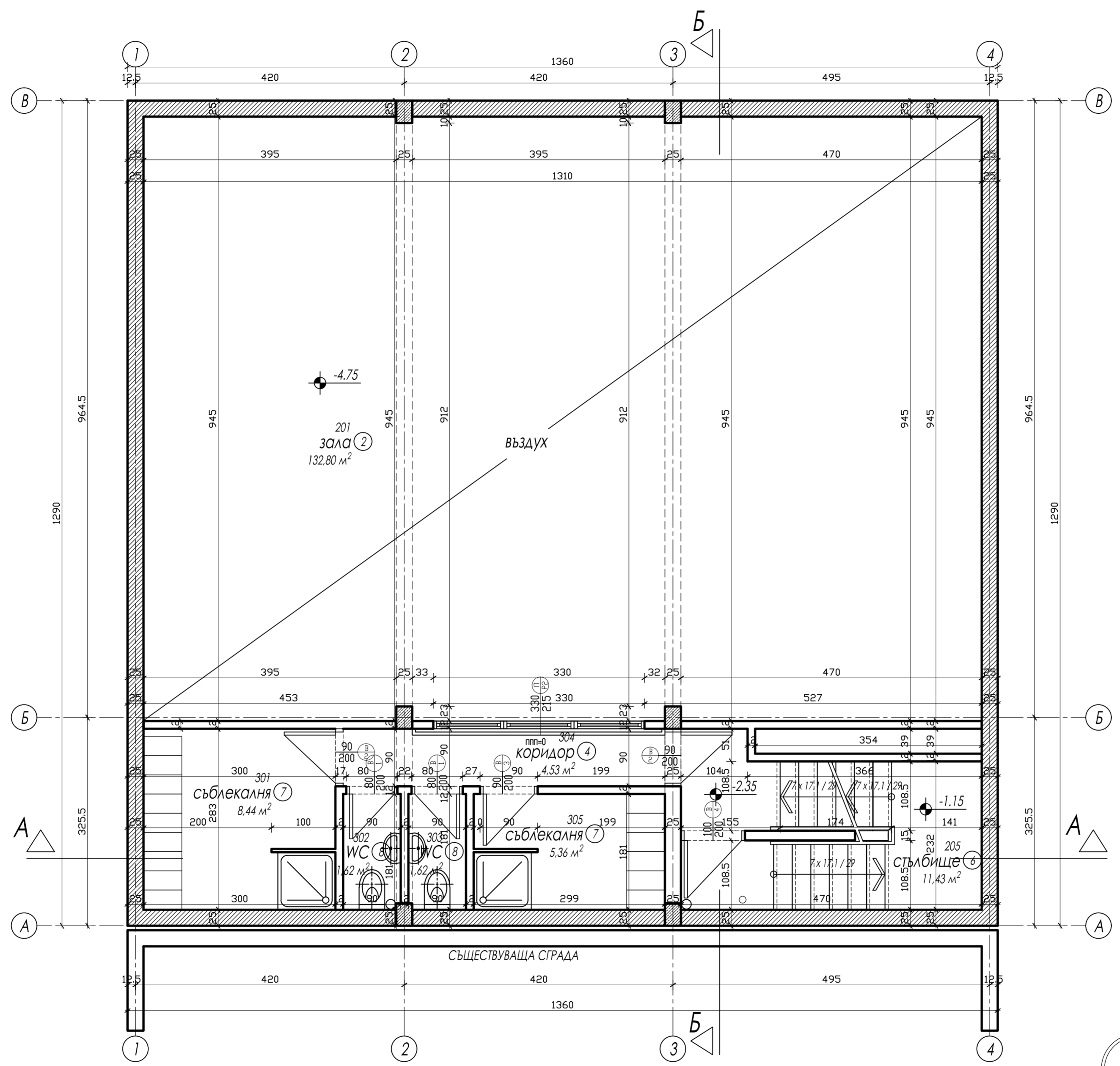
РАЗПРЕДЕЛЕНИЕ КОТА -2,35
